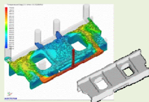
鋳造湯流れ・凝固解析
